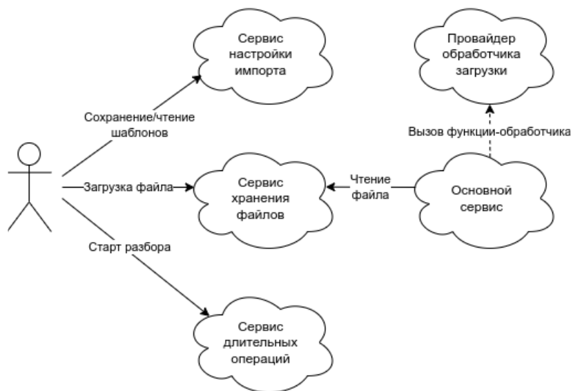
Рисунок 1. Схема взаимодействия сервисов
